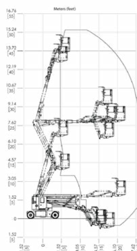
ENVELOPPE DE TRAVAIL SJ45 AJN
