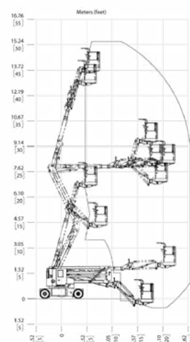
ENVELOPPE DE TRAVAIL SJ45 ARJN
