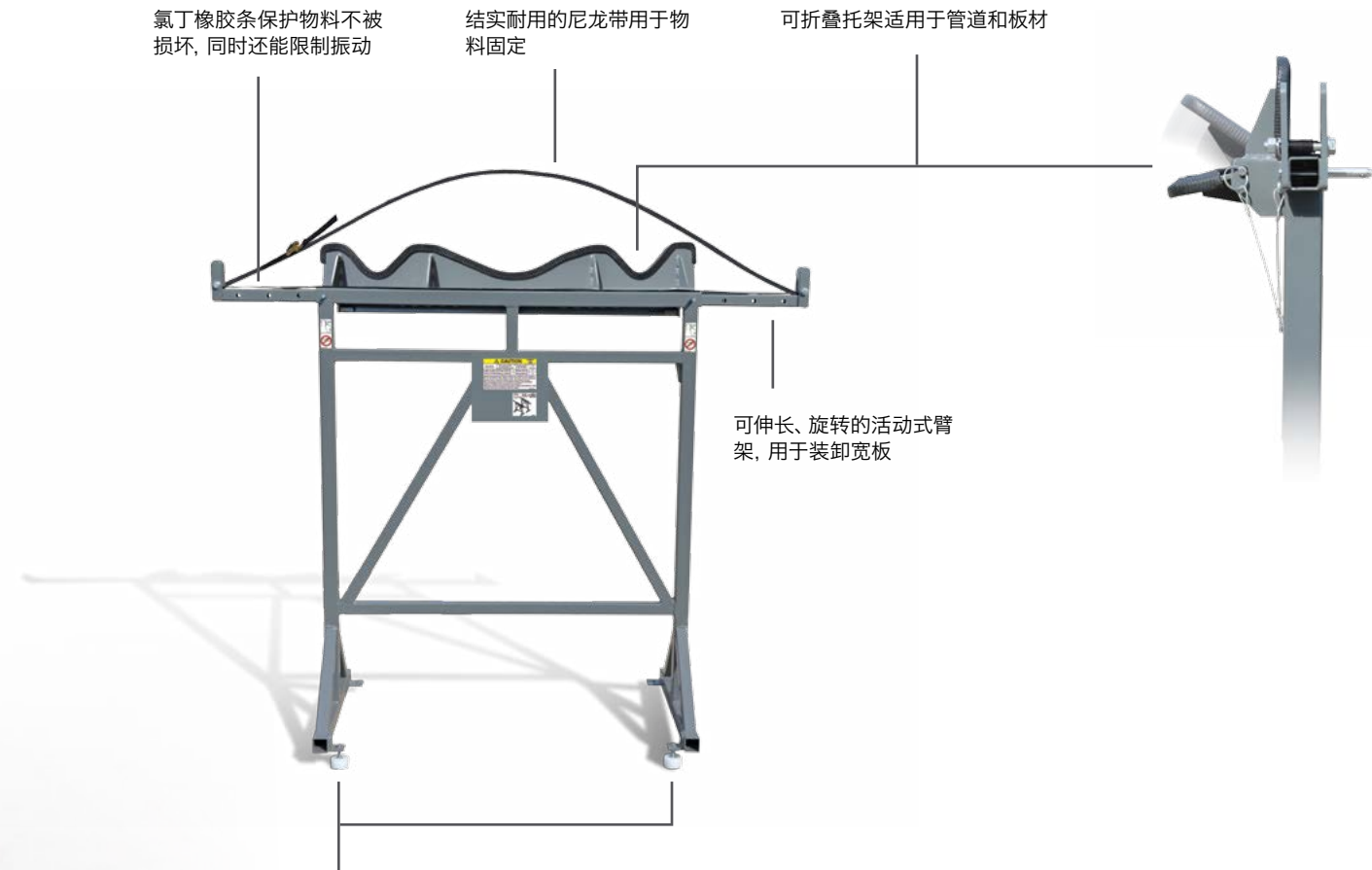
当装置安装在平台延伸台面固定端而橡胶压轮安装在主台面上时，橡胶压轮可使台面自由伸缩
